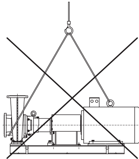
Рис. 4 Неправильный способ строповки насоса
