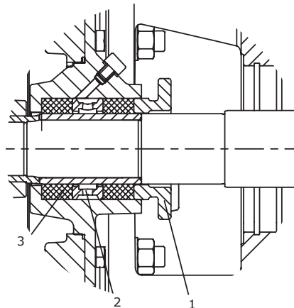
Рис. 24 Сальниковая бокса в разрезе
